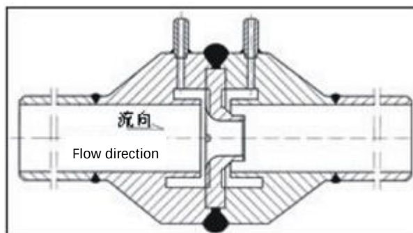
A: ISA 1932 nozzle
